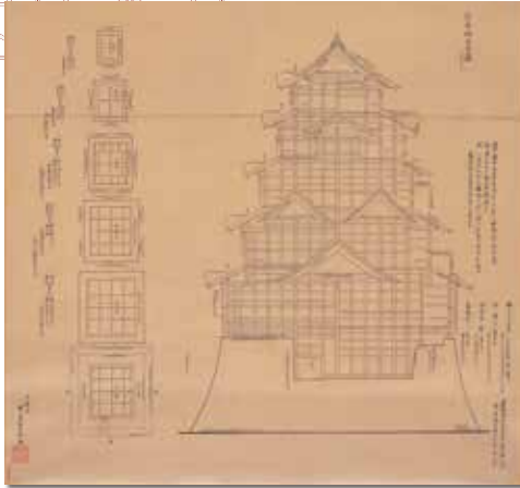
重要文化財 江戸城御本丸御天守 1/100 建地割
